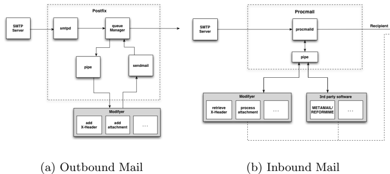
Fig. 1. Archiving Using SMTP
